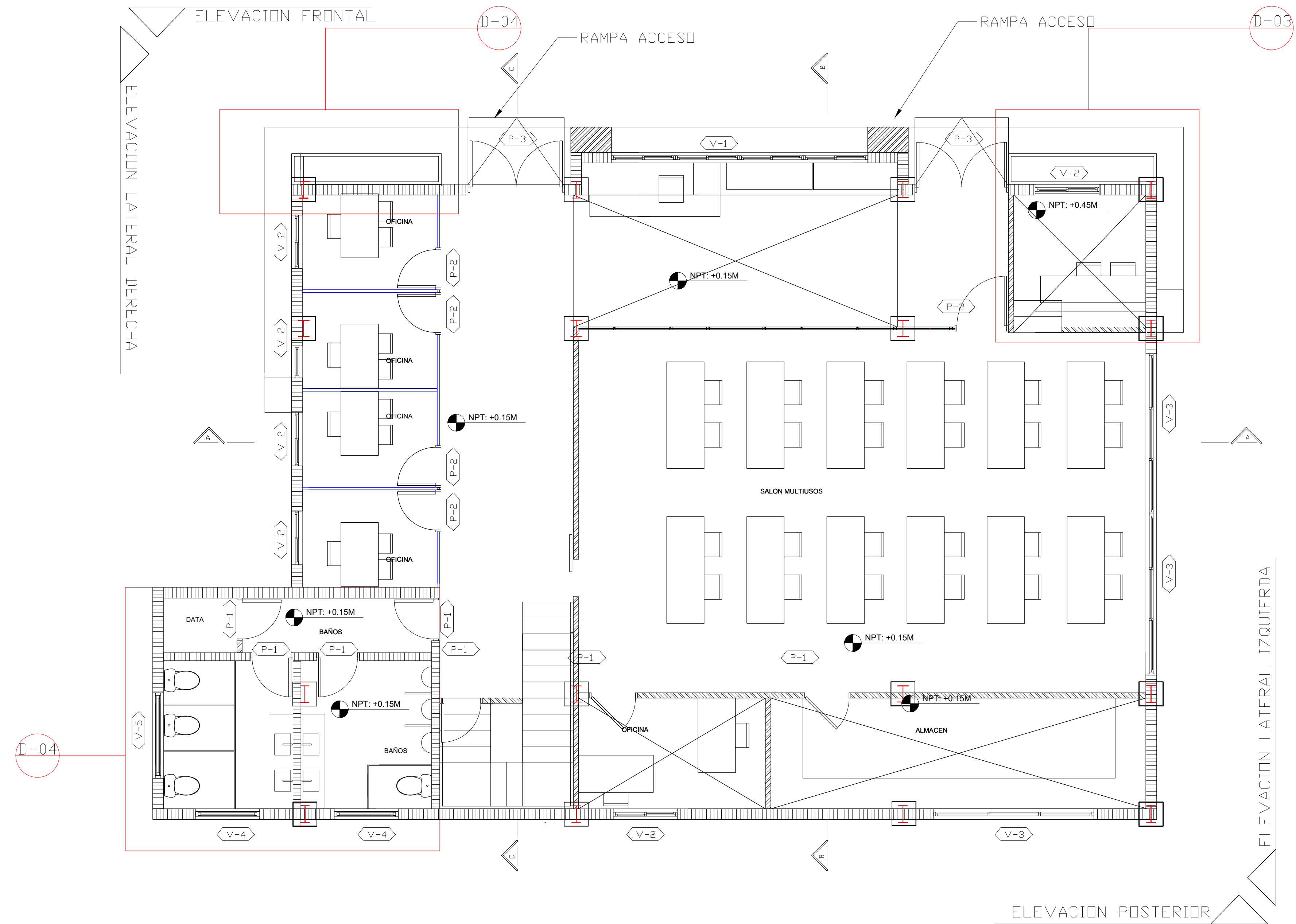
[01 PLANTA ARQUITECTONICA AMUEBLADA PRIMER NIVEL
